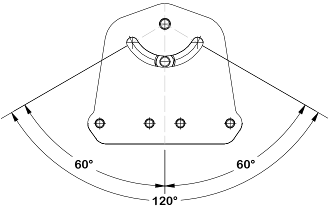
PIVOT RANGE
